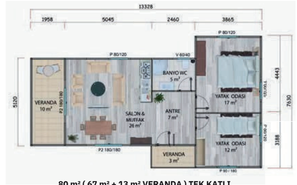
80 m 2 ( 67 m 2 + 13 m 2 VERANDA ) TEK KATLI PREFABRİK KONUT PLANI
