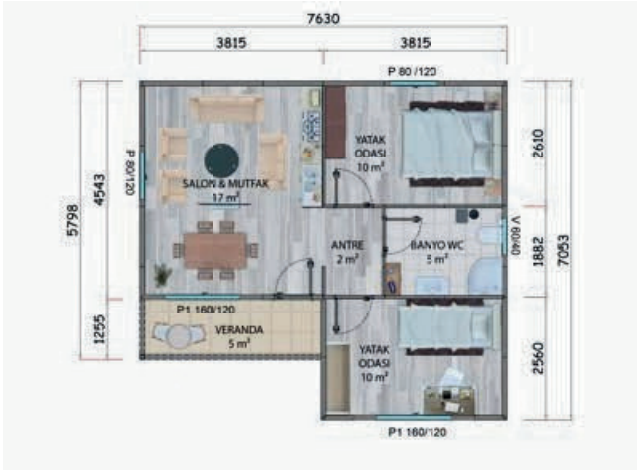
49 m 2 ( 44 m 2 + 5 m 2 VERANDA ) TEK KATLI PREFABRİK KONUT PLANI
