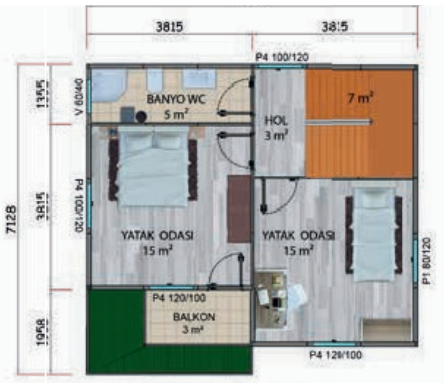
48 m 2 (45 m 2 + 3 m 2 BALKON) 1. KAT PLANI
