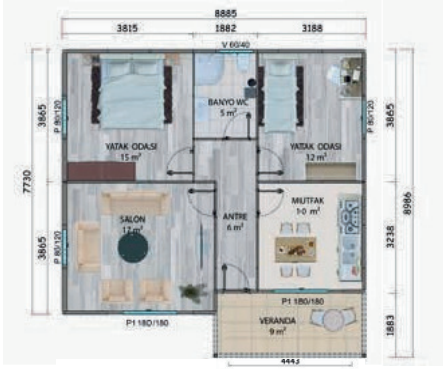
74 m 2 ( 65 m 2 + 9 m 2 VERANDA ) TEK KATLI PREFABRİK KONUT PLANI
