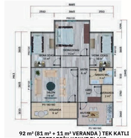
92 m 2 ( 81 m 2 + 11 m 2 VERANDA ) TEK KATLI PREFABRİK KONUT PLANI
